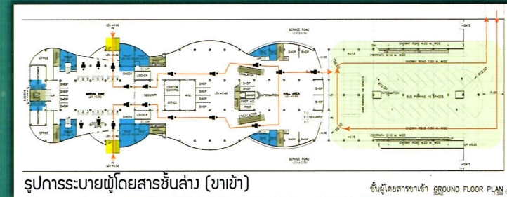
ชั้นผู้โดยสารขาเข้า GROUND FLOOR PLAN
